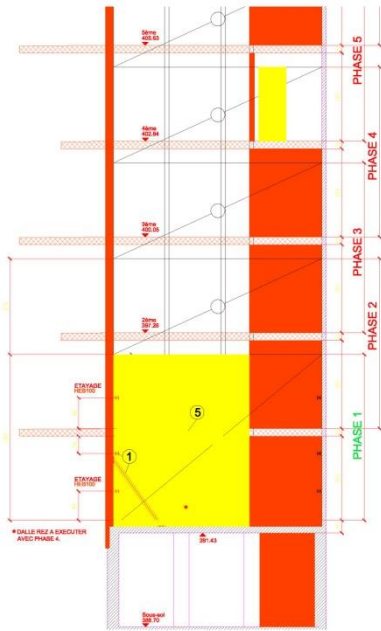
Coupe verticale – phases des travaux
